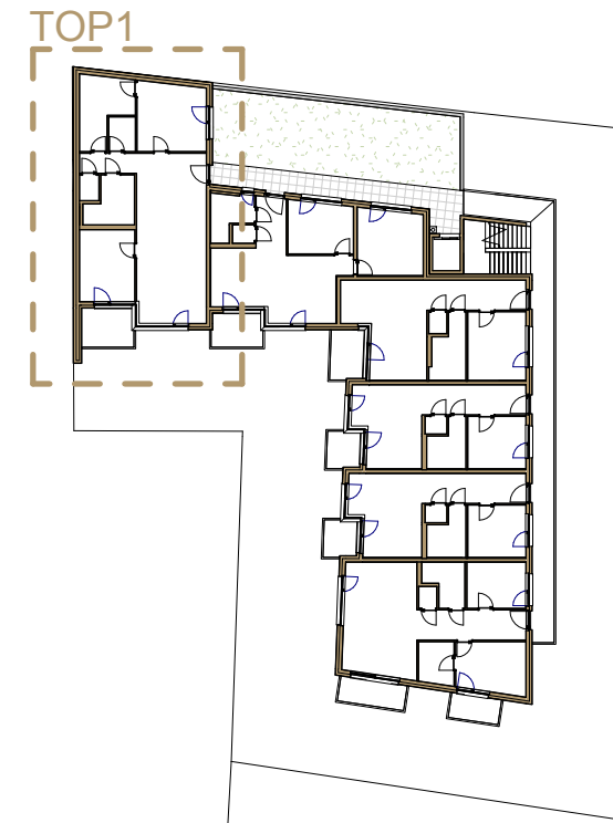
2 1.Obergeschoß 1 : 500
