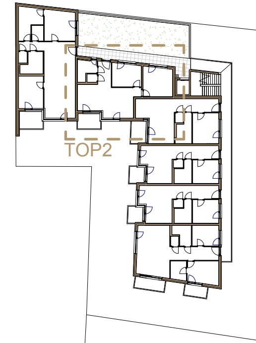
2 1.Obergeschoß 1 : 500
