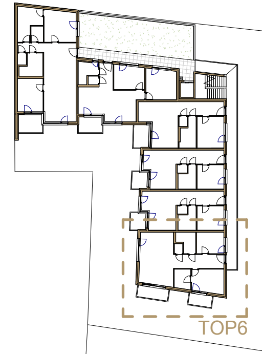
2 1.Obergeschoß 1 : 500
