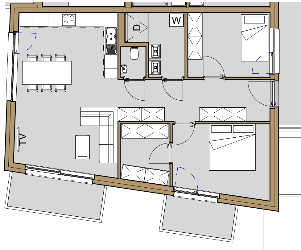
1 TOP6 1 : 100
