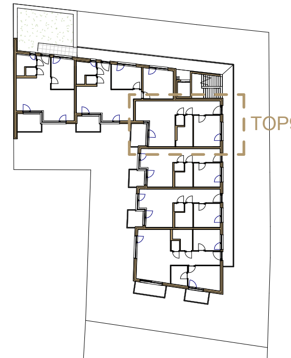
2 2.Obergeschoß 1 : 500
