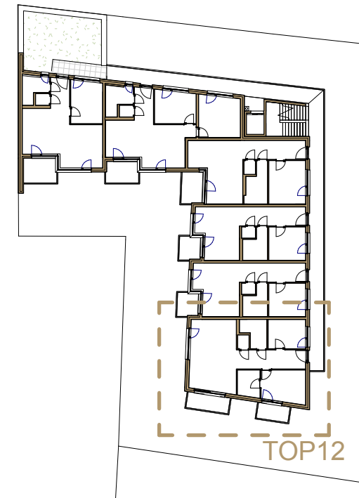
2 2.Obergeschoß 1 : 500
