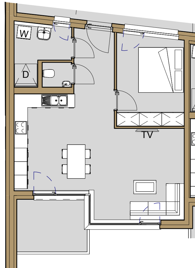
1 TOP13 1 : 100
