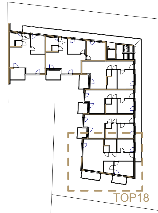
2 3.Obergeschoß 1 : 500
