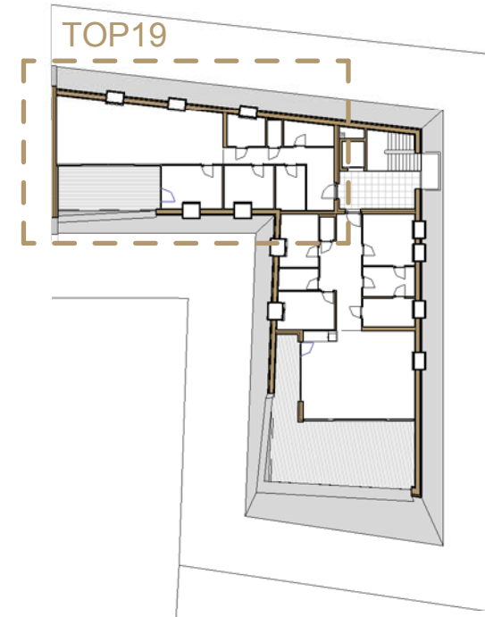
2 Dachgeschoß 1 : 500
