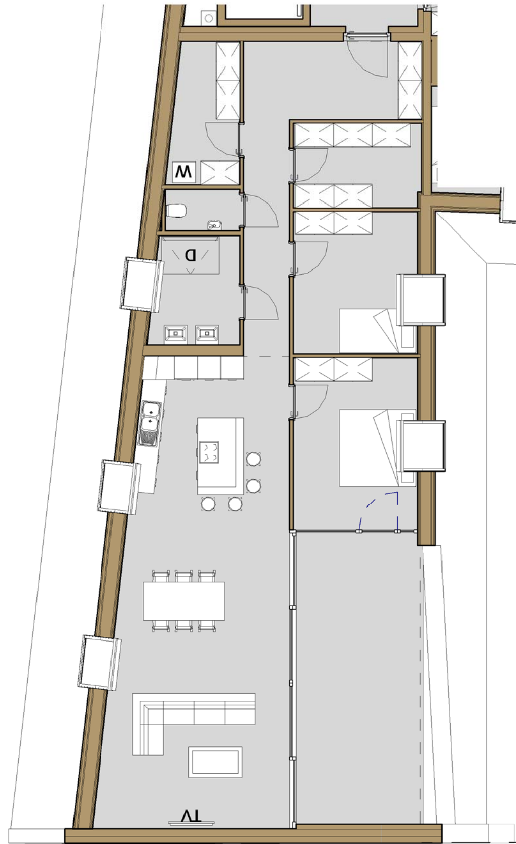
1 TOP19 1 : 100
